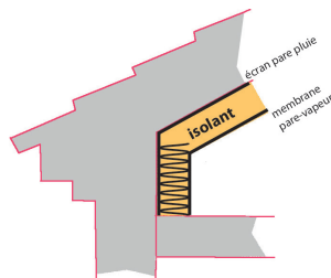
Comble habité
