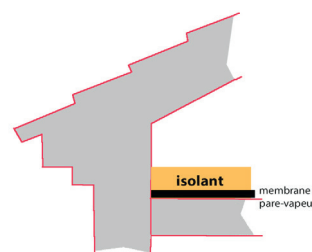
Comble perdu
