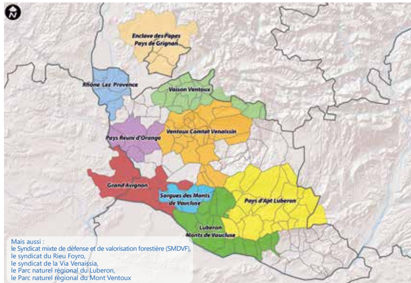
Intercommunalités adhérentes en 2021
