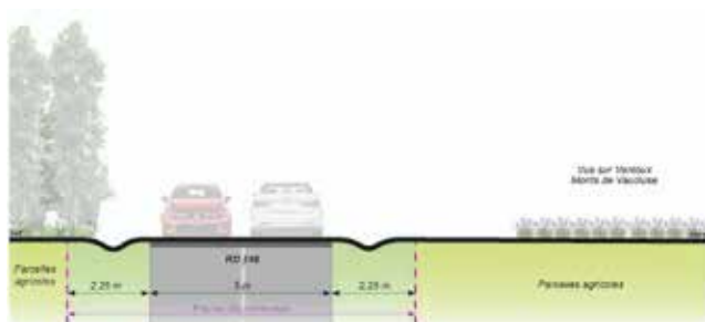
ETAT EXISTANT - PROFIL DE PRINCIPLE
